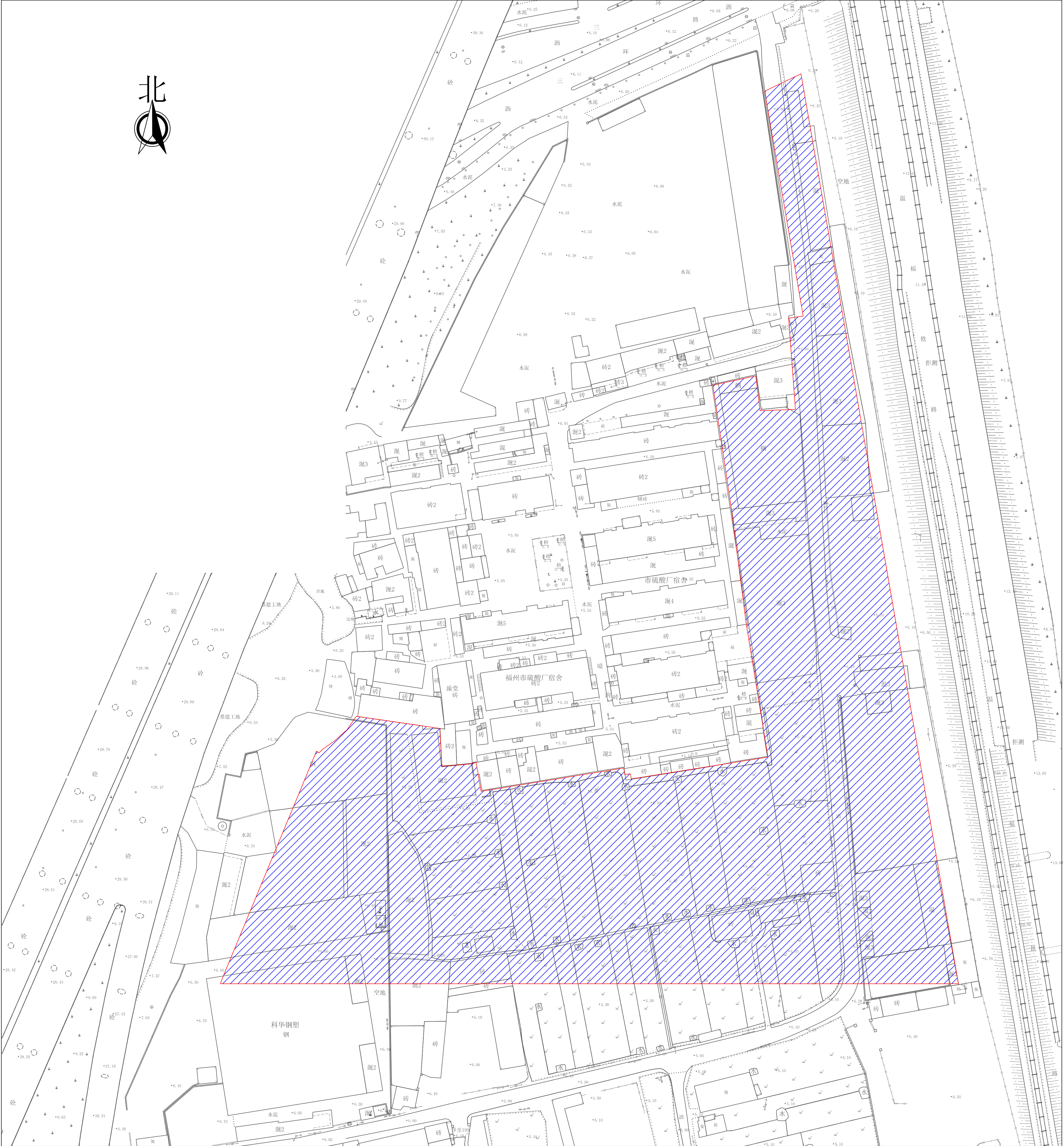
原福州洋里污水处理厂及配套管网三期工程棚户区改造地块规划选址红线图
