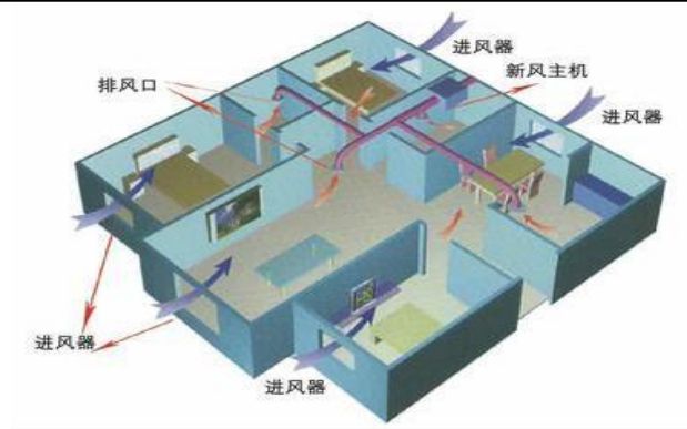
图 4-2 新风系统原理示意图
