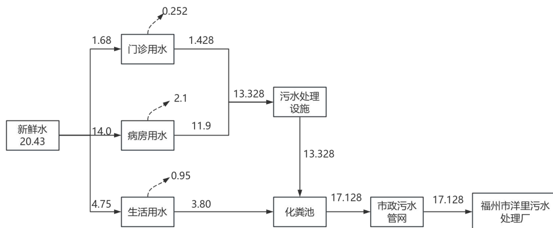
图 2.6-1 扩建项目水平衡 单位： \text{m}^3/\text{d}
