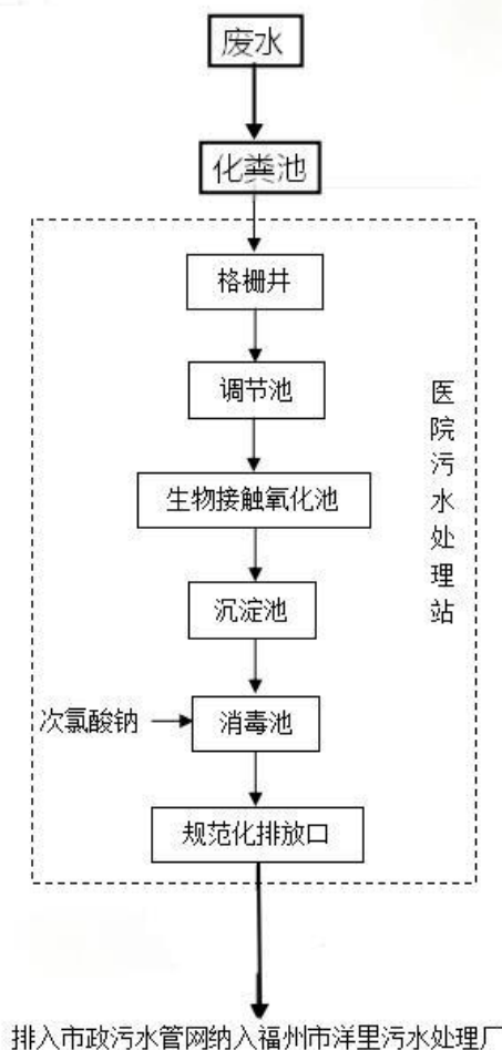
图 4.3-1 污水处理工艺流程图
